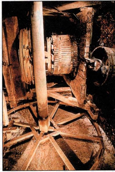
Pressoir à roue de perroquet
