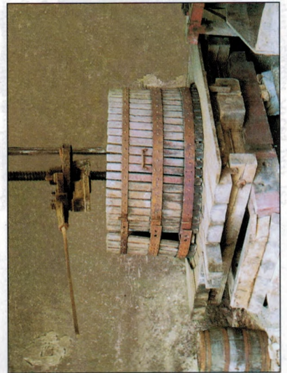
Pressoir à cliquet ou à barre.
